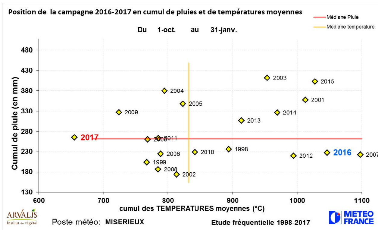
Figures 5 à 8 : Position de la campagne 2016-2017 en cumul de pluies et de températures moyennes pour différents postes météo
